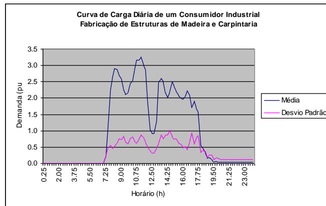
Figura 3 – Exemplo de curva de carga típica de consumidor industrial
