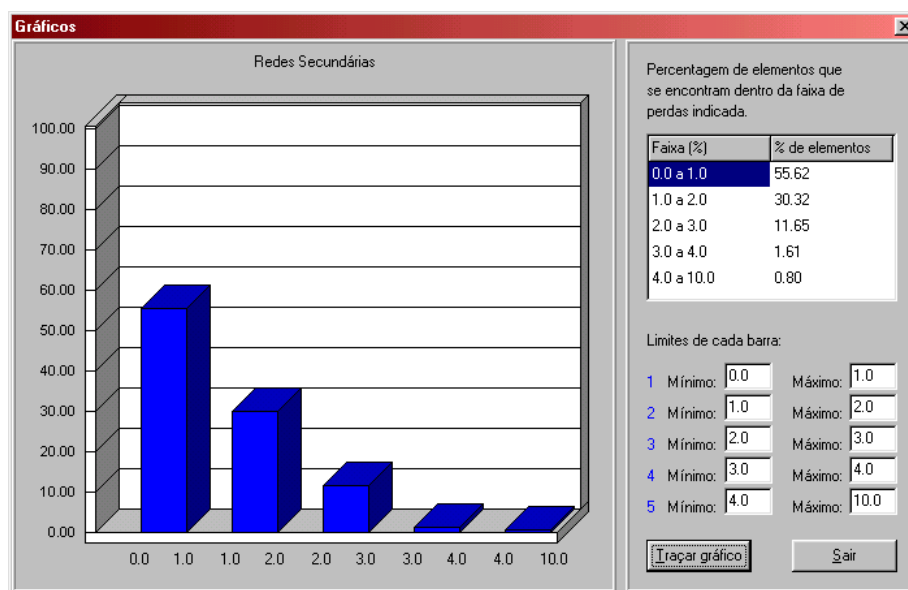
Figura 9 – Histograma da perda de energia no segmento rede secundária
