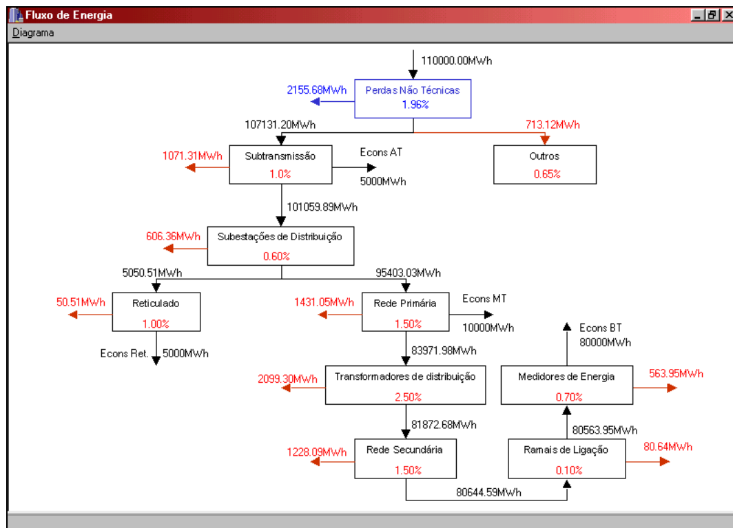
Figura 11 – Diagrama do fluxo de energia no sistema de distribuição
