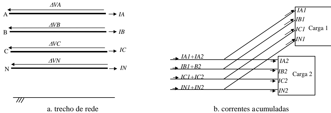
Figura 4 – Rede secundária
