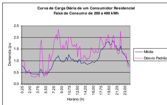
Figura 2 – Exemplo de curva de carga típica de consumidor residencial
